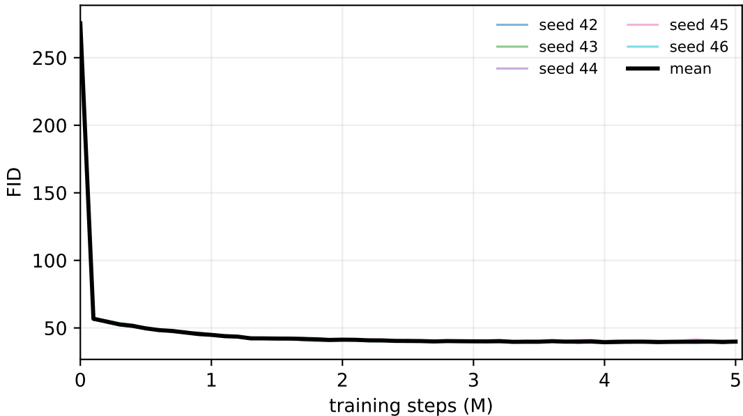
CelebA d=80
